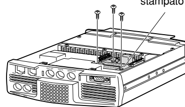
Filtro IF/ scheda a circuito stampato TCXO
